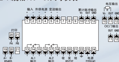
■ A规格160×80尺寸仪表
