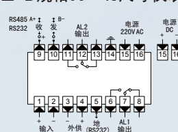
■ D规格96×48尺寸仪表
